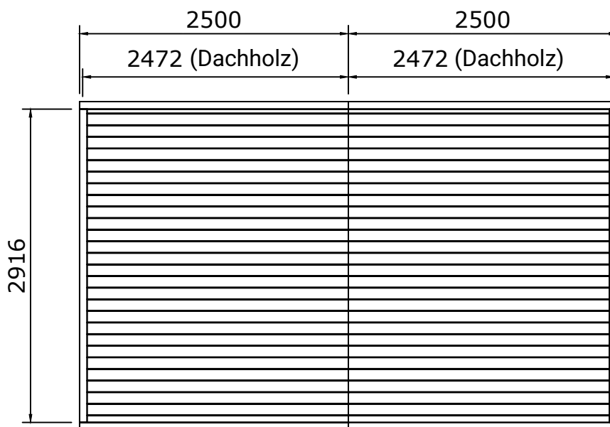
Obenansicht
